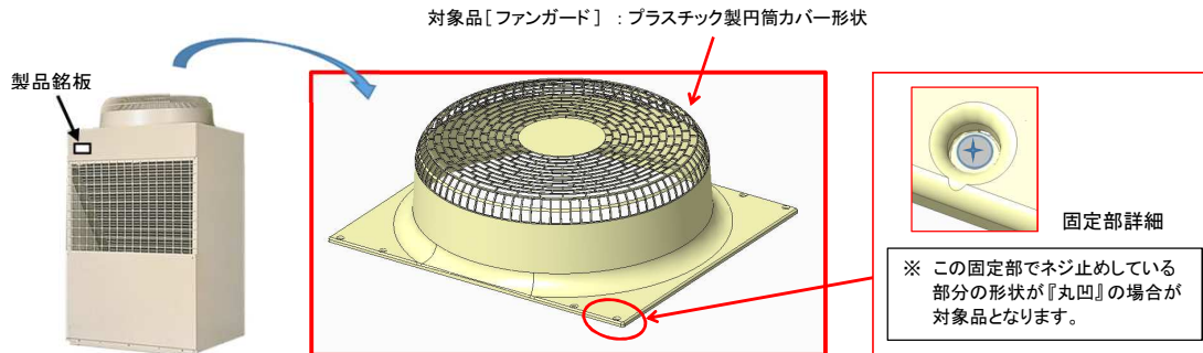
図1. 外観
